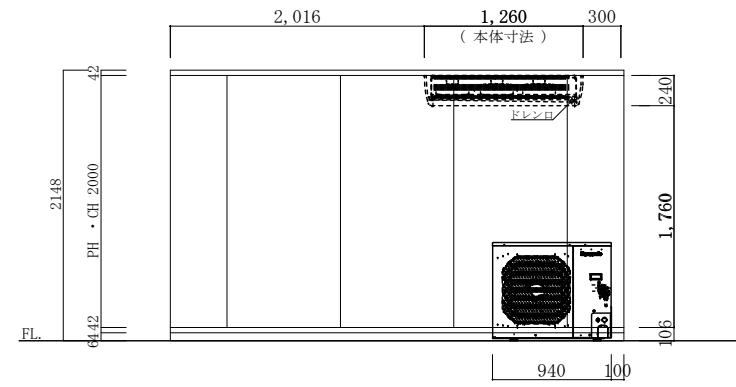
立面図B
