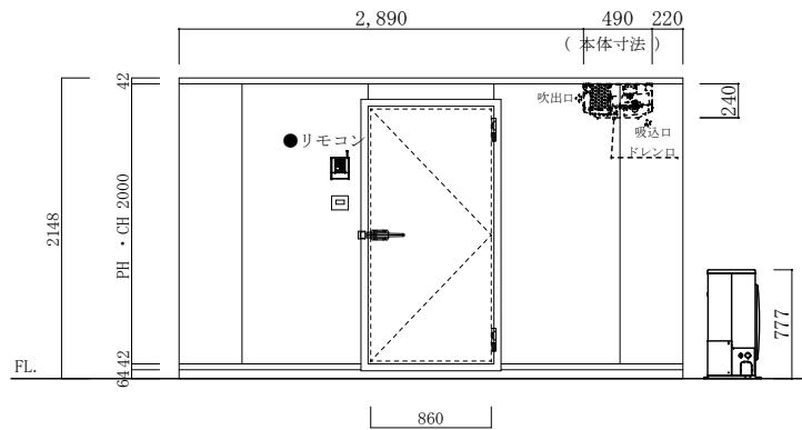
立面図A
