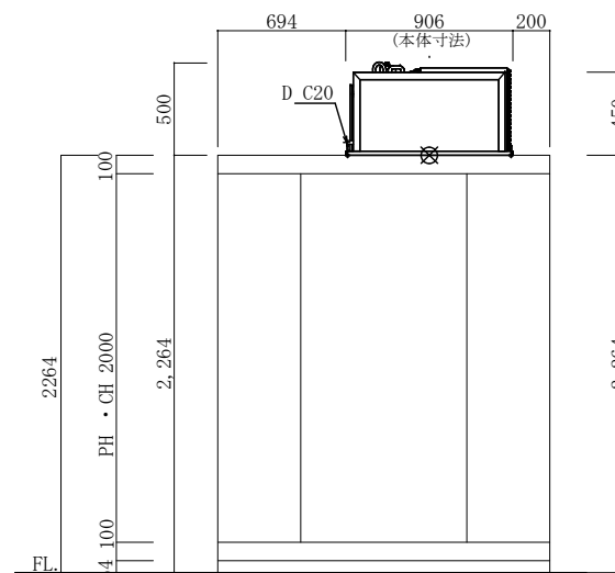
立面図B
