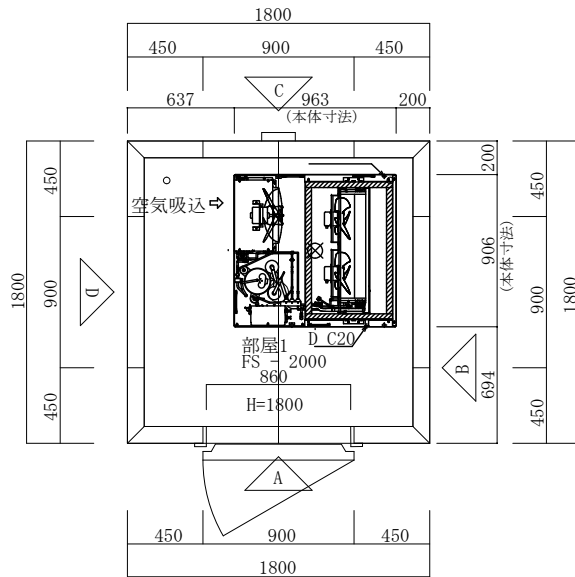
平面図
