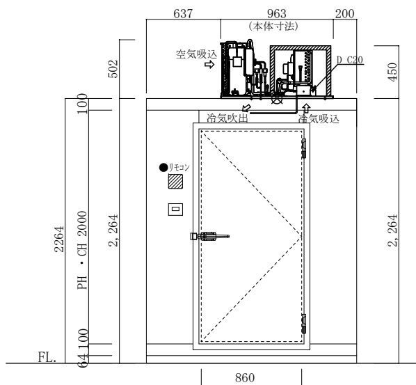
立面図A
