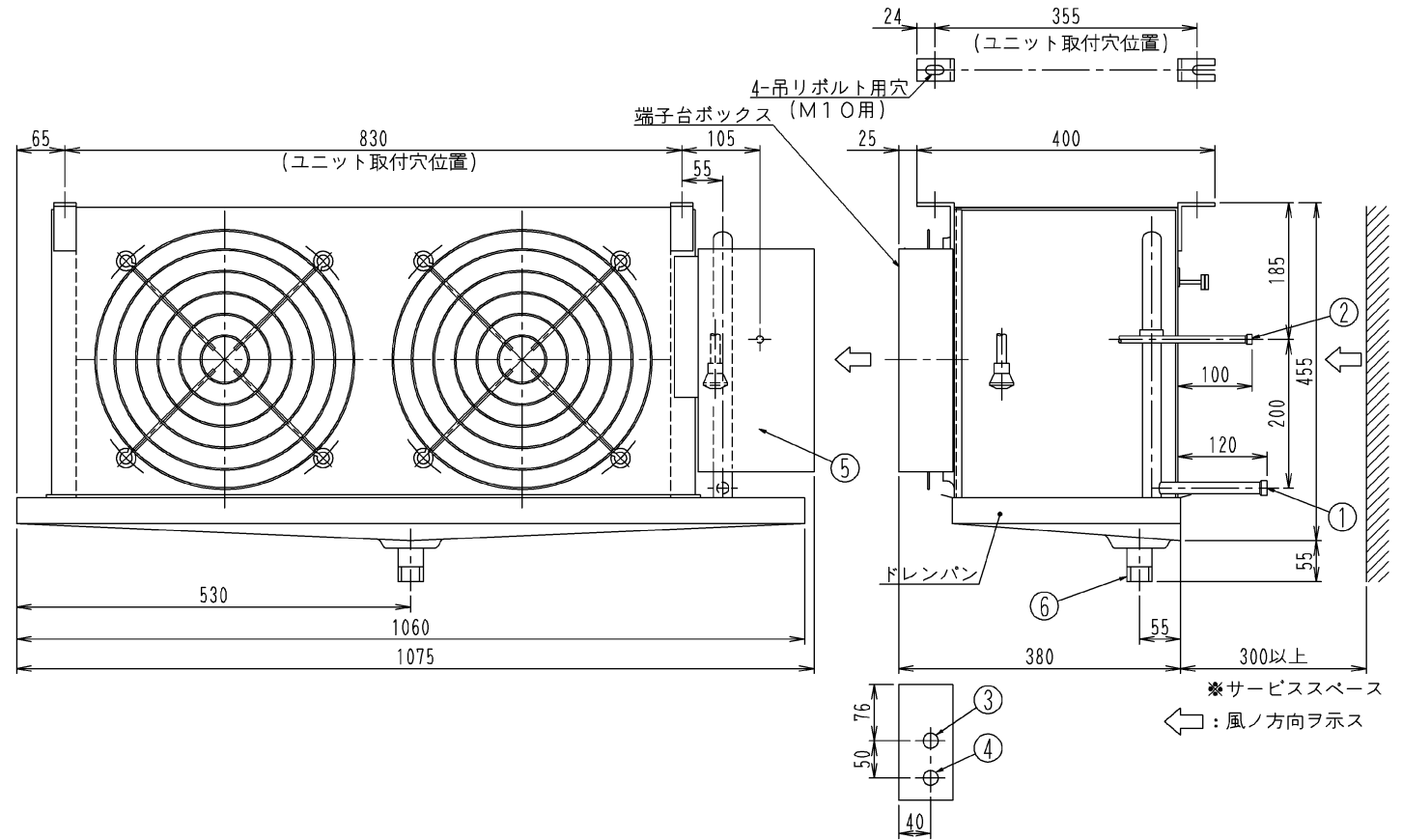
端子台ボックス下面図 (連絡配線取出口詳細)
