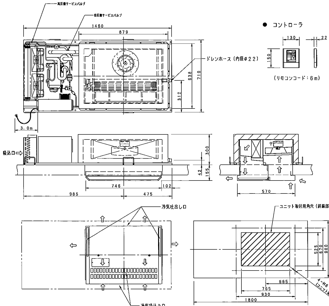
ユニット取付寸法図
