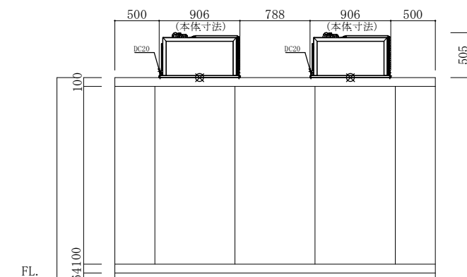
立面图B
