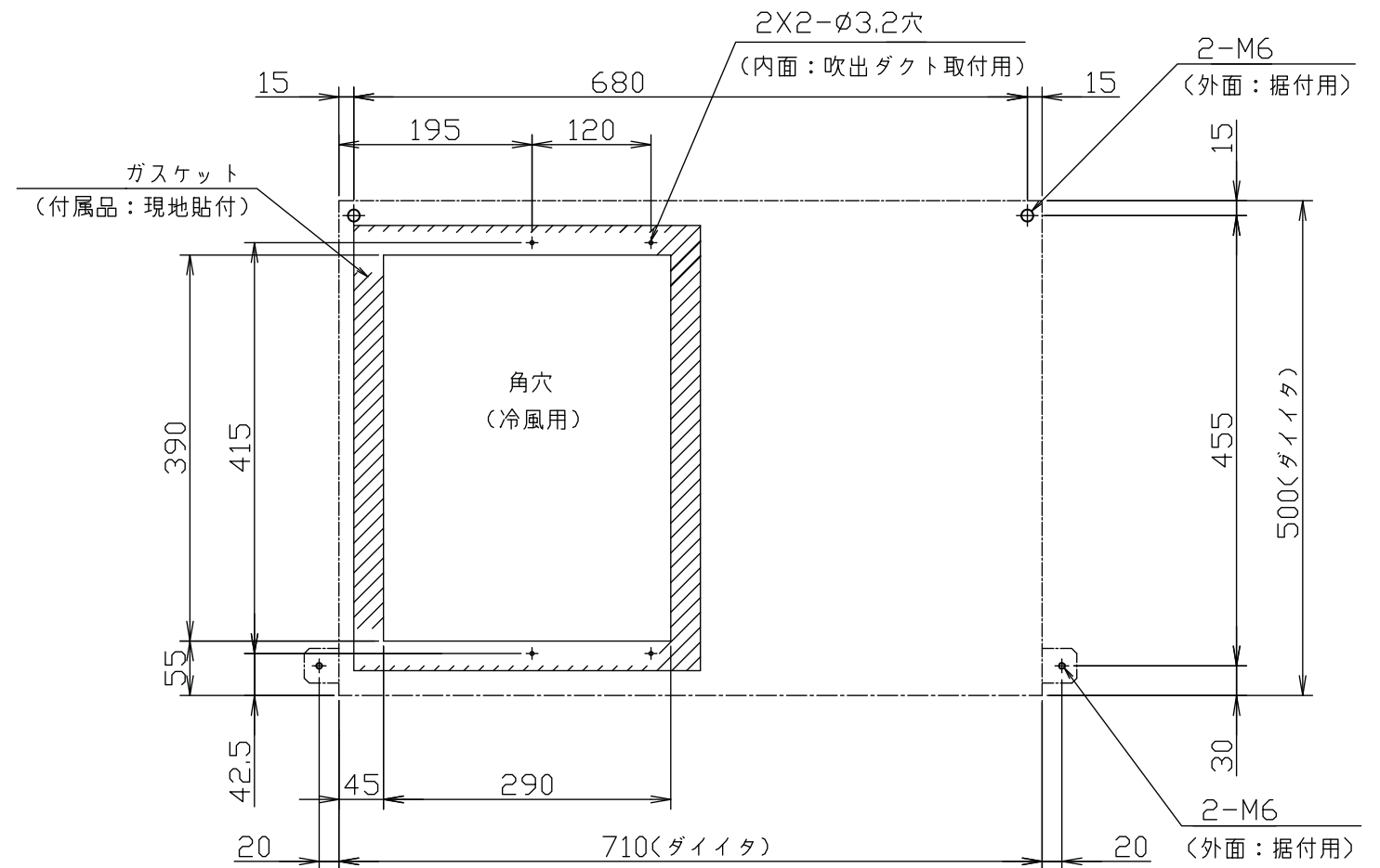
据付寸法図
