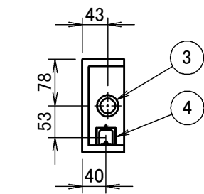
電気品箱下面図 (連絡配線取出口詳細)
