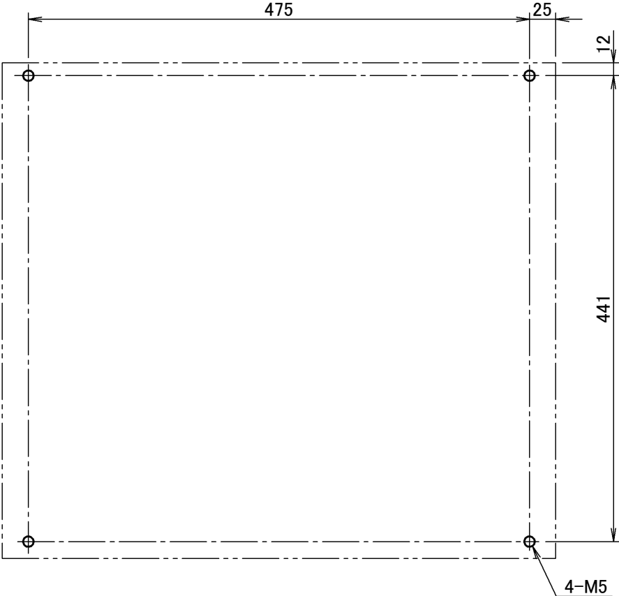
取付穴位置 (正面図)
